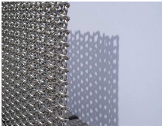
Materiaal: GOLF SIERRA small transparantie bij loodrechte stand materiaal; minder doorlaat
