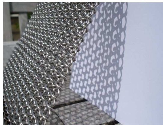
Materiaal: GOLF SIERRA small transparantie bij schuine stand materiaal, resulteert in grotere doorlaat
